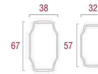
profilo bracci "tipo A" "A" type arms profile
